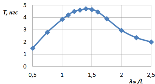
Рис. 7. Резонанс размерной тяги ВГ на встречном волнении ( \beta=180 ). Параметры: v_0 = 2 узла; \bar{x}_{тр}=0 ; S_{\Sigma\text{кр}} = S_{\text{гвл}} ; \bar{L}_{тр}=46 .
