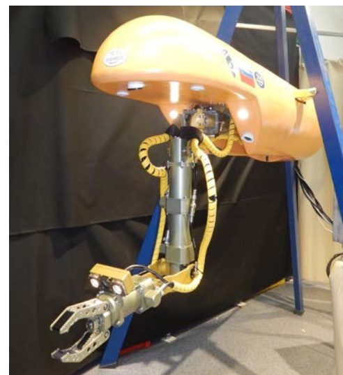
Стенд-манипулятор версии 2.2
